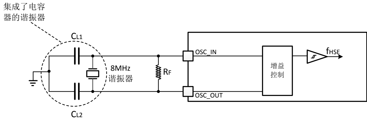
图11. 控制模块使用8 ~ 24MHz晶体的典型应用
