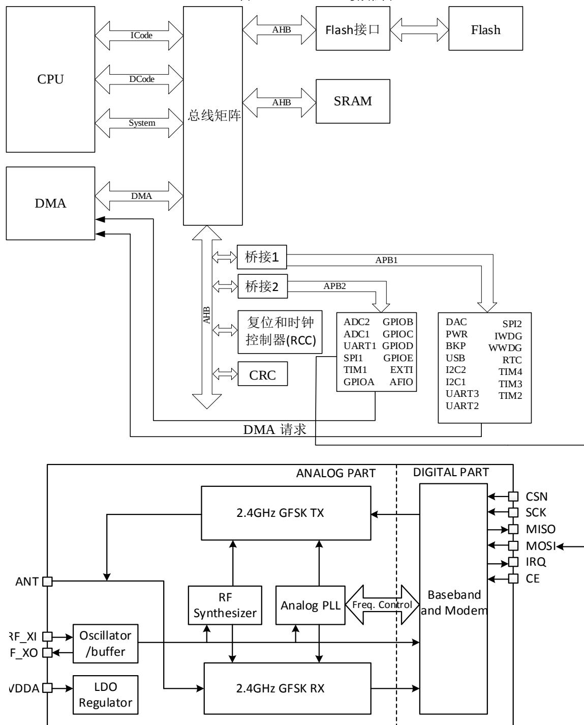
图1. MM32W3x2xxB模块框图
