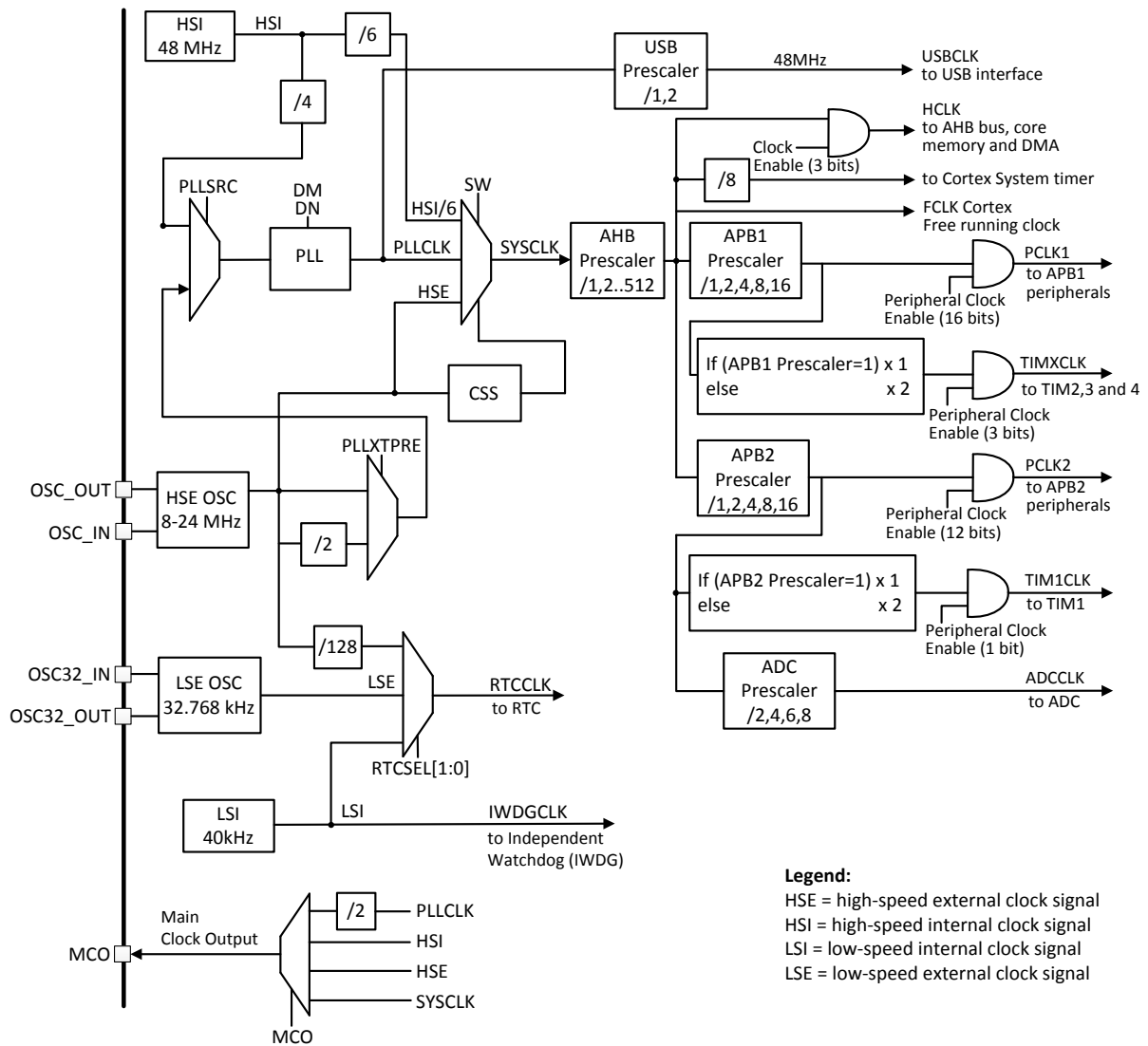
图 2. 时钟树
