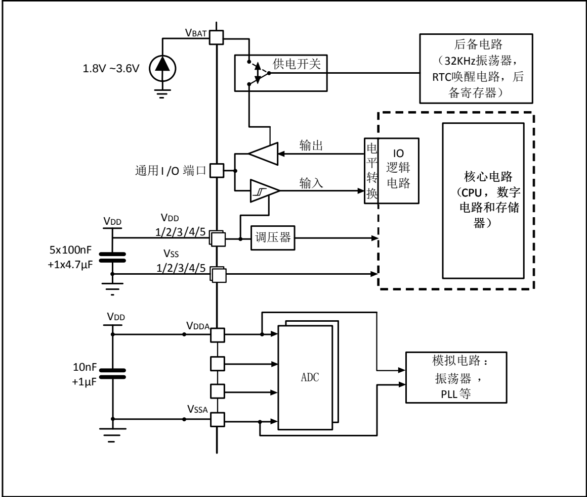
图 7. 供电方案
