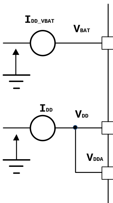
图 8. 电流消耗测量方案
